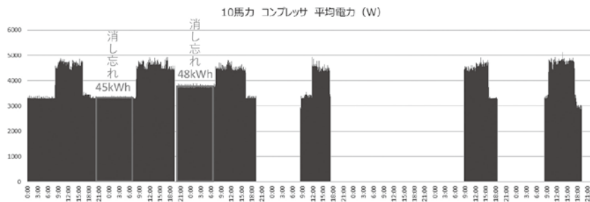
〈省エネ診断を行った工場でのコンプレッサの電力消費計測結果(1週間)〉
